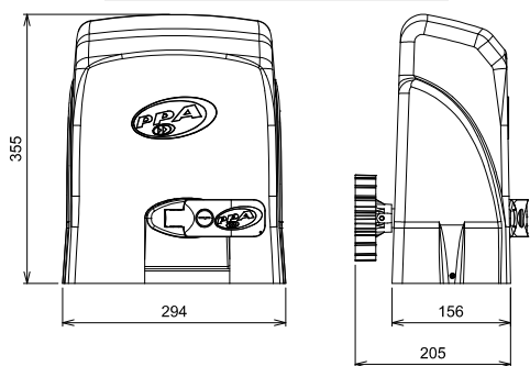
DIMENSÕES DO EQUIPAMENTO
